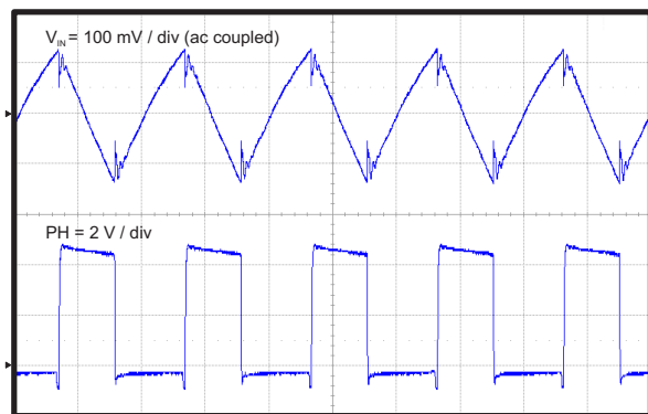
INPUT RIPPLE, I_{OUT} = 7 A
