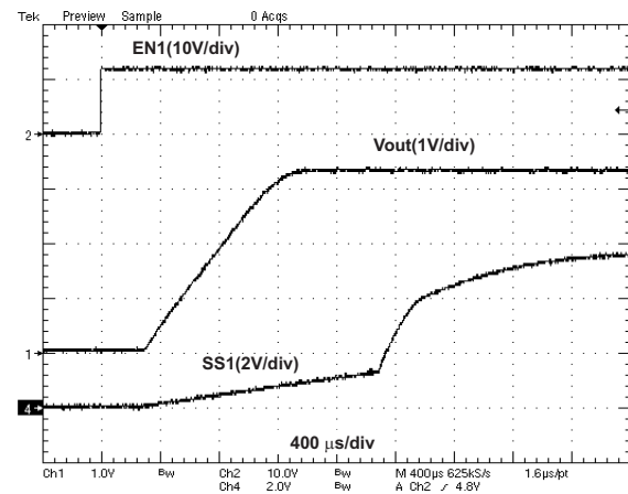
Figure 10. VO1=3.3V, SoftStart
