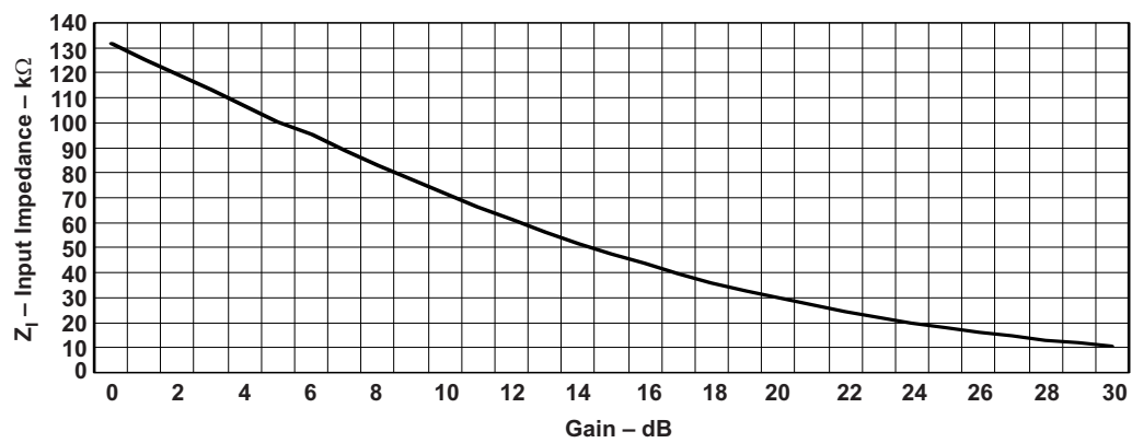
Figure 28. Nominal Input Impedance - Per Leg
