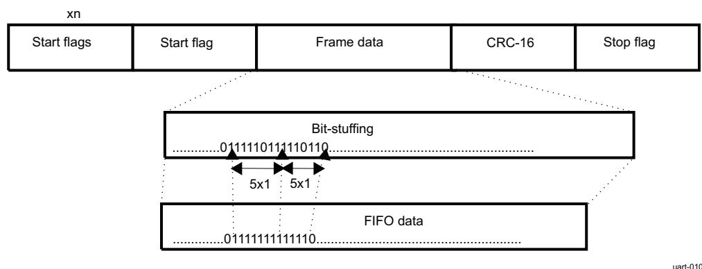
Figure 23-8. MIR Transmit Frame Format
