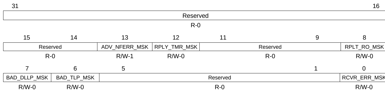
Figure 17-121. PCIE_CERR_MASK Register
