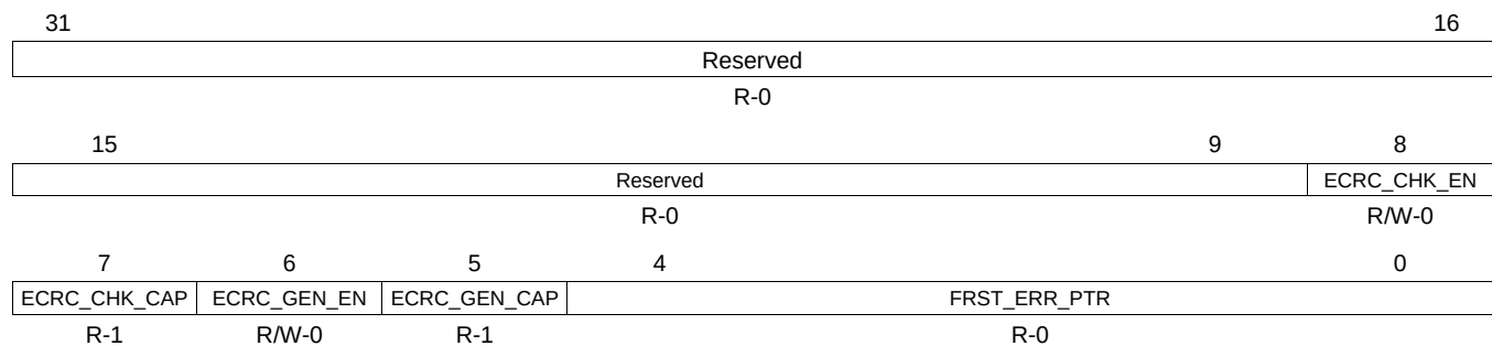
Figure 17-122. PCIE_ACCR Register
