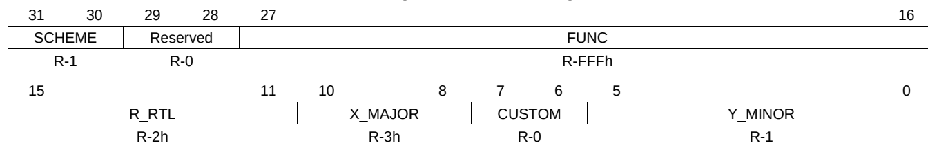
Figure 21-8. TIDR Register
