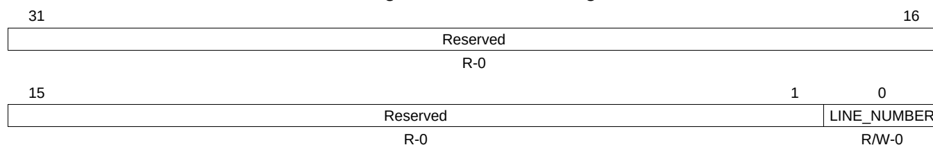
Figure 8-9. GPIO_EOI Register
