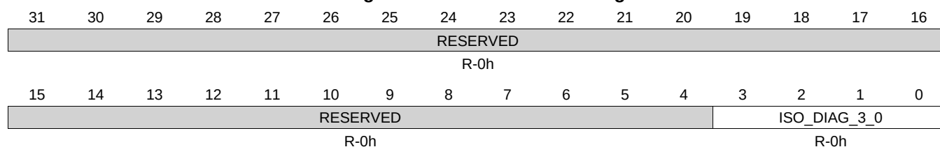
Figure 3-21. ISODIAGSTAT Register
