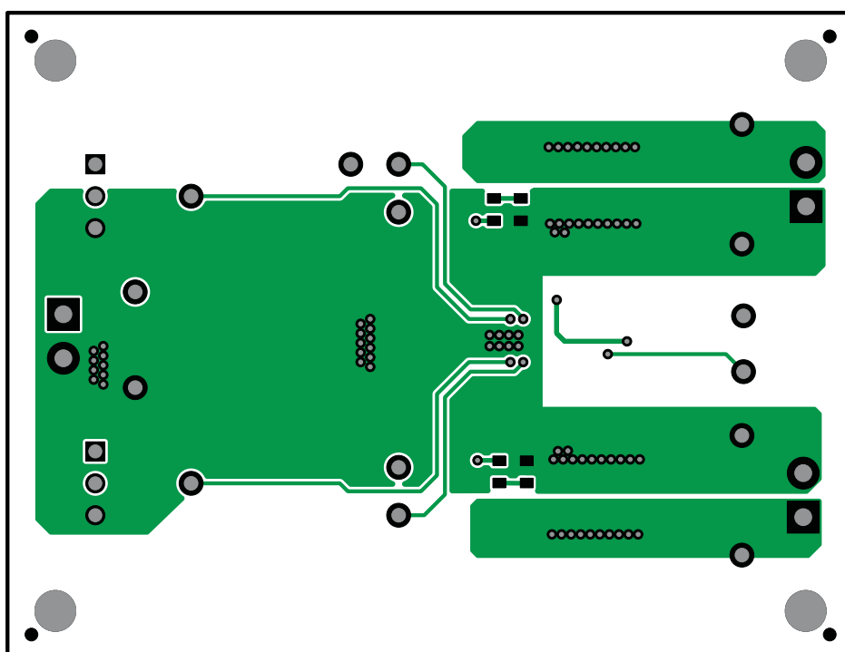
Figure 24. Bottom Layer
