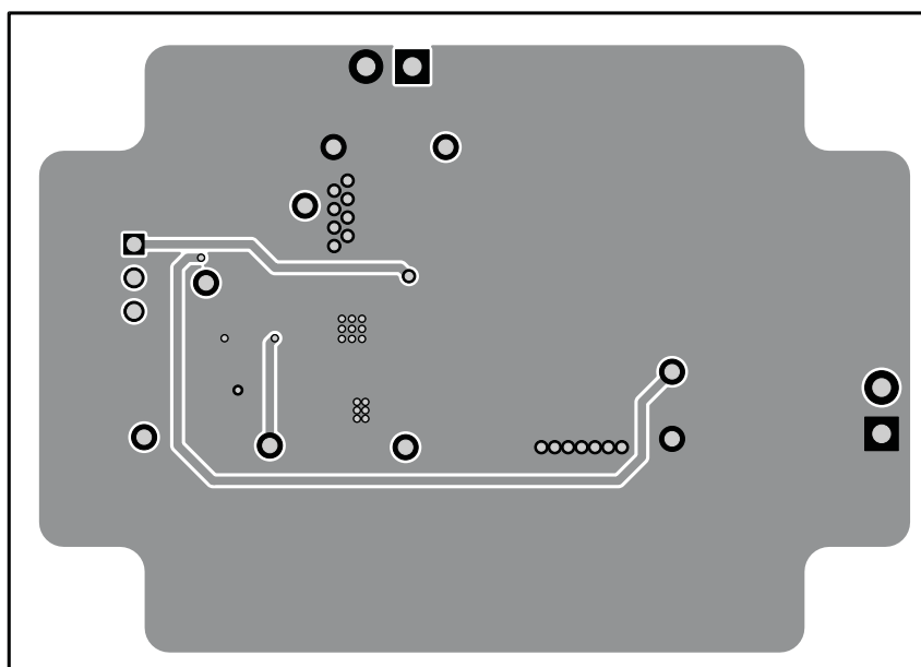
Figure 20. Bottom Layer
