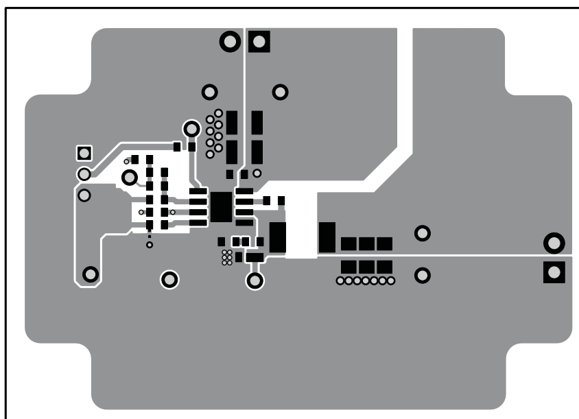
Figure 17. Top Layer
