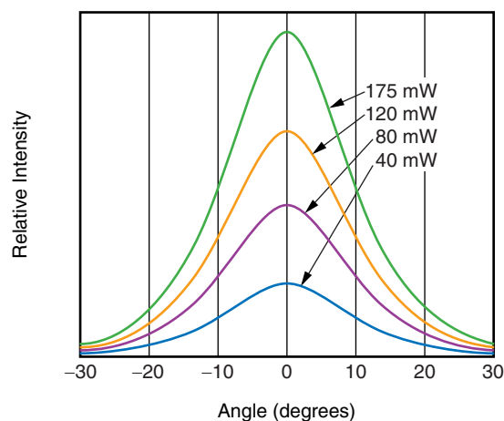
FFP (VERTICAL)
