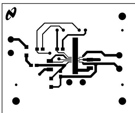
Top Layer
