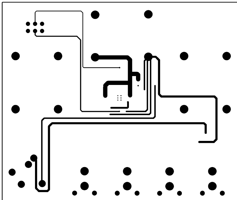
Figure 47. Bottom Layer
