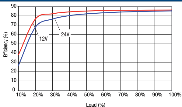
NCS6S4803C
