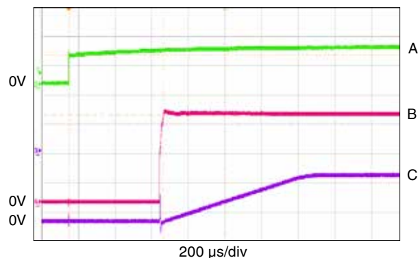
Enable Waveform
