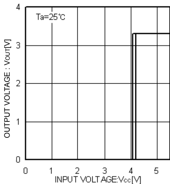
Fig.4 Vcc-Vout
