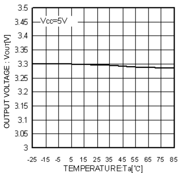
Fig.7 Ta-Vout
