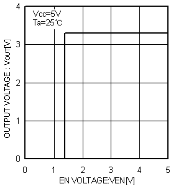
Fig.5 Ven-Vout
