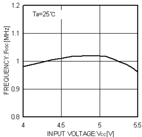
Fig.13 V_{cc} - F_{osc}
