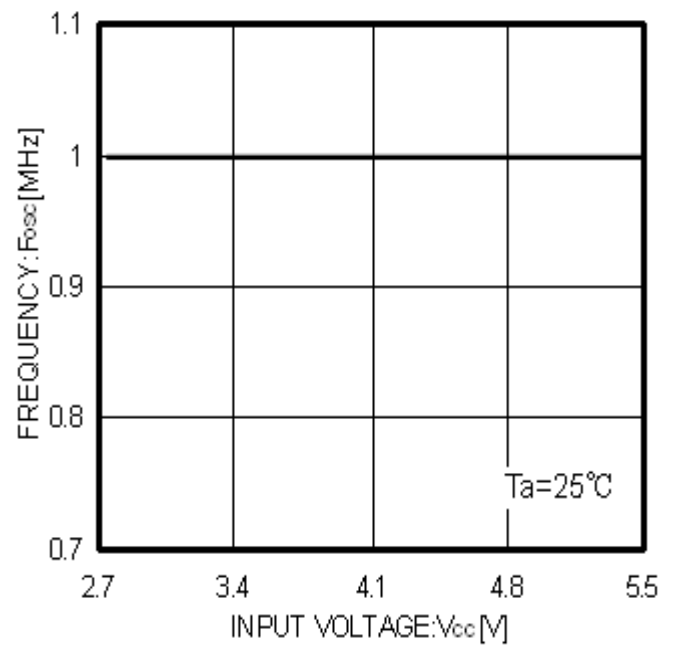
Fig.13 V_{cc} - F_{osc}
