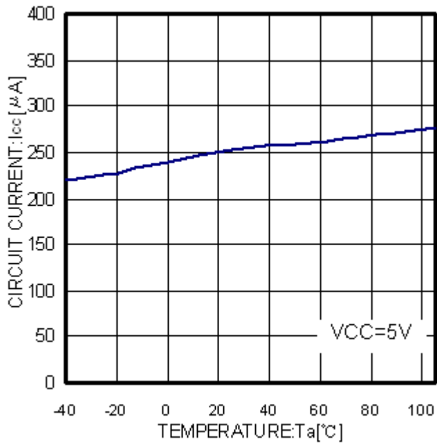
Fig.12 T_a - I_{cc}
