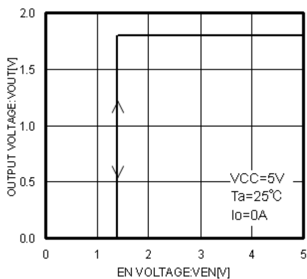
Fig.5 Ven-Vout
