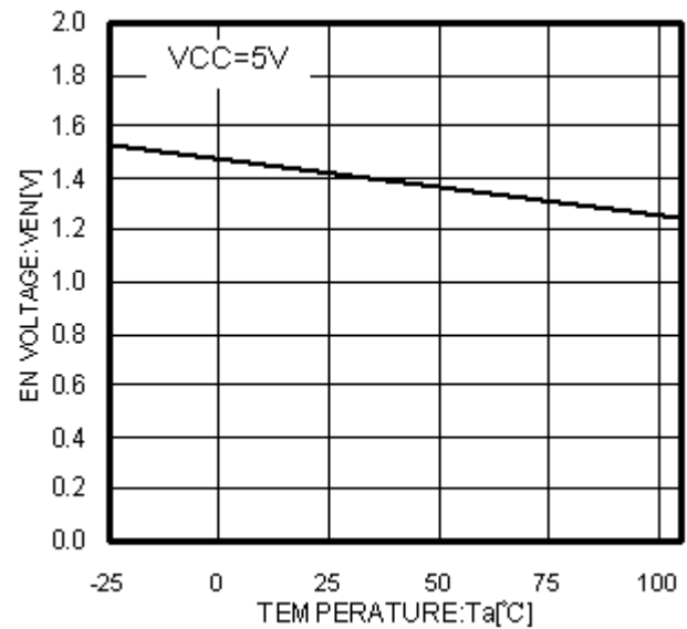
Fig.11 Ta-VEN
