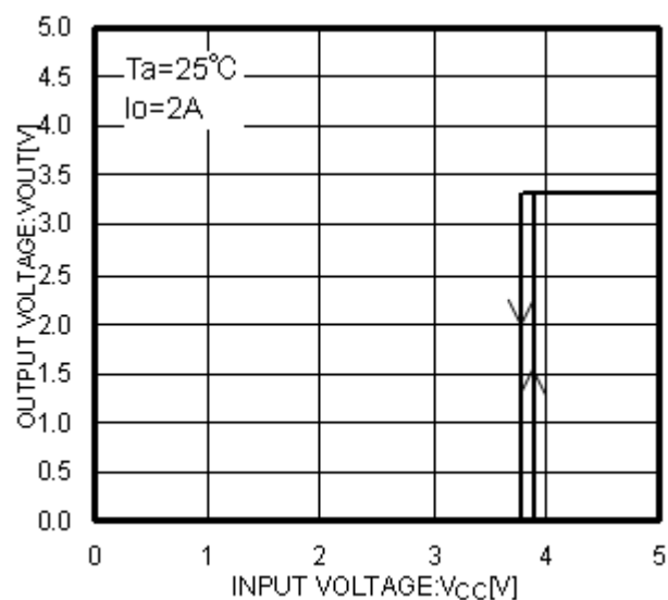
Fig.4 Vcc-Vout
