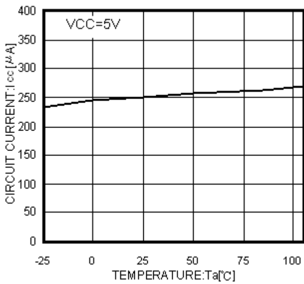
Fig.12 T_a - I_{cc}
