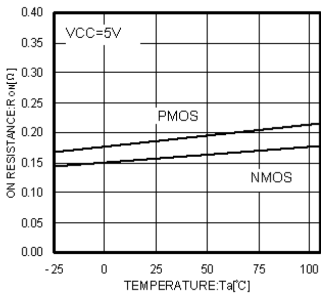
Fig.10 Ta-RONN, RONP
