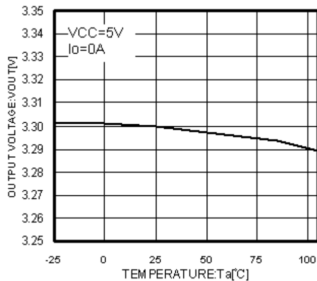
Fig.7 Ta-Vout
