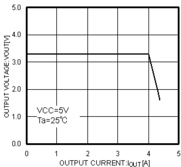
Fig.6 Iout-Vout
