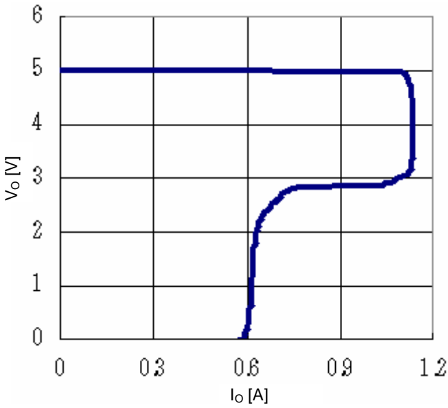
Fig.16 OCP
