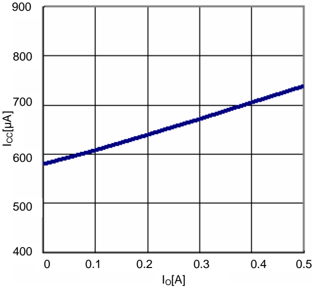
Fig.19 I_o - I_{cc}
