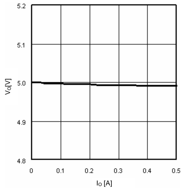
Fig.12 Io-Vo
