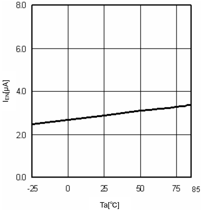
Fig.11 Ta-IEN
