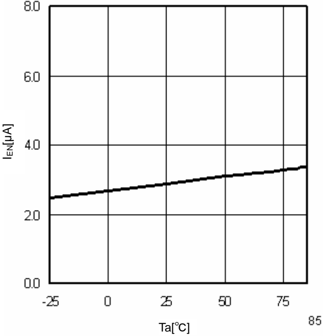
Fig.11 T_a - I_{EN}
