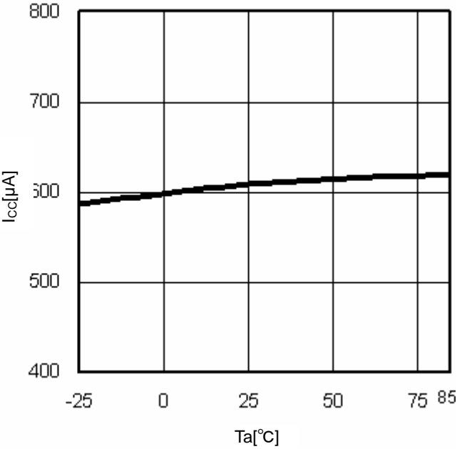
Fig.9 T_a-I_{CC}
