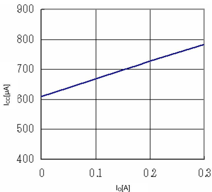
Fig.19 I_o - I_{cc}
