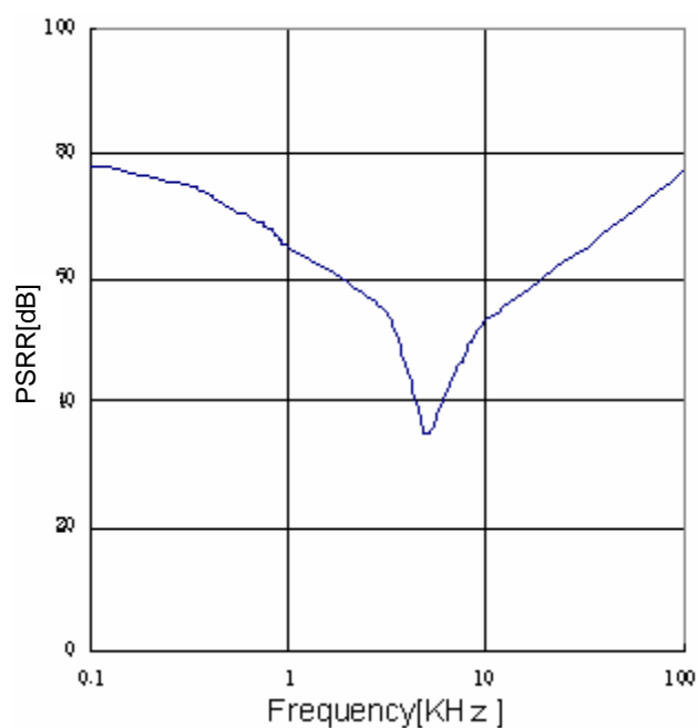
Fig.20 PSRR( I_o=0mA )
