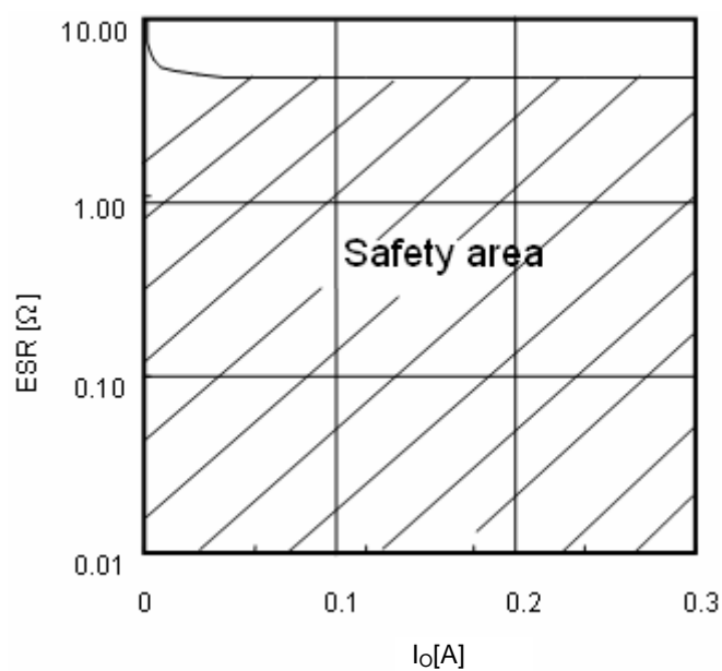
Fig.18 ESR condenser
