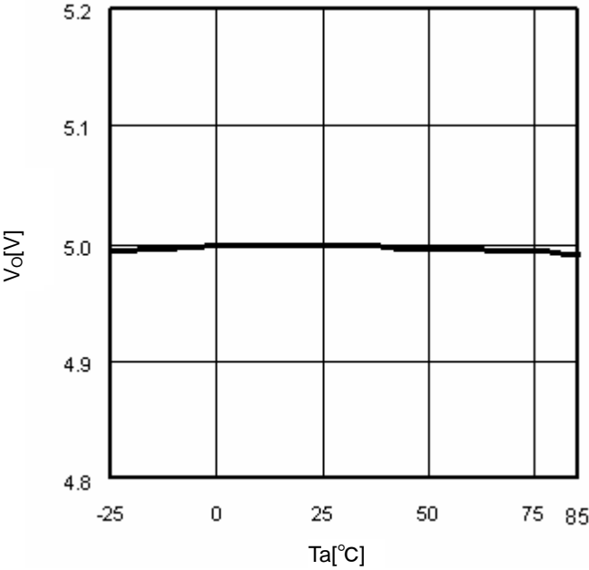
Fig.8 T_a-V_O ( I_O=0mA )
