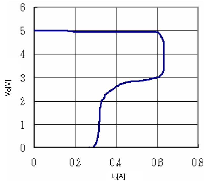
Fig.16 OCP
