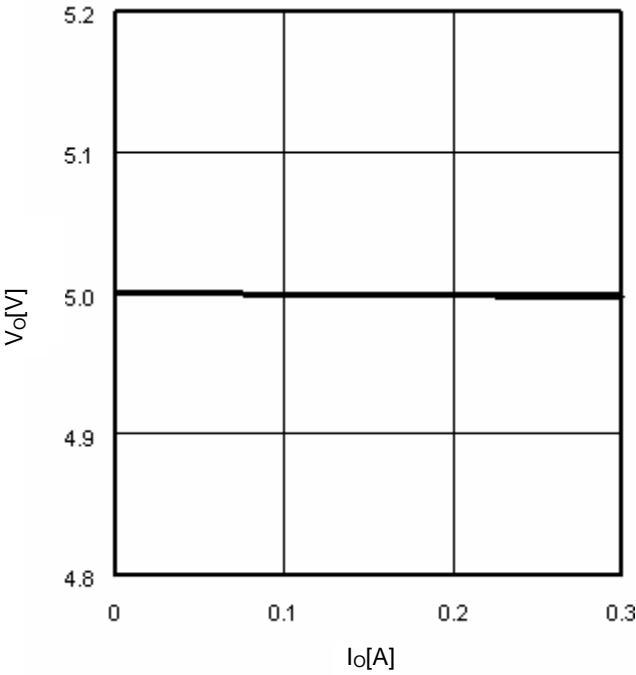
Fig.12 I_o - V_o
