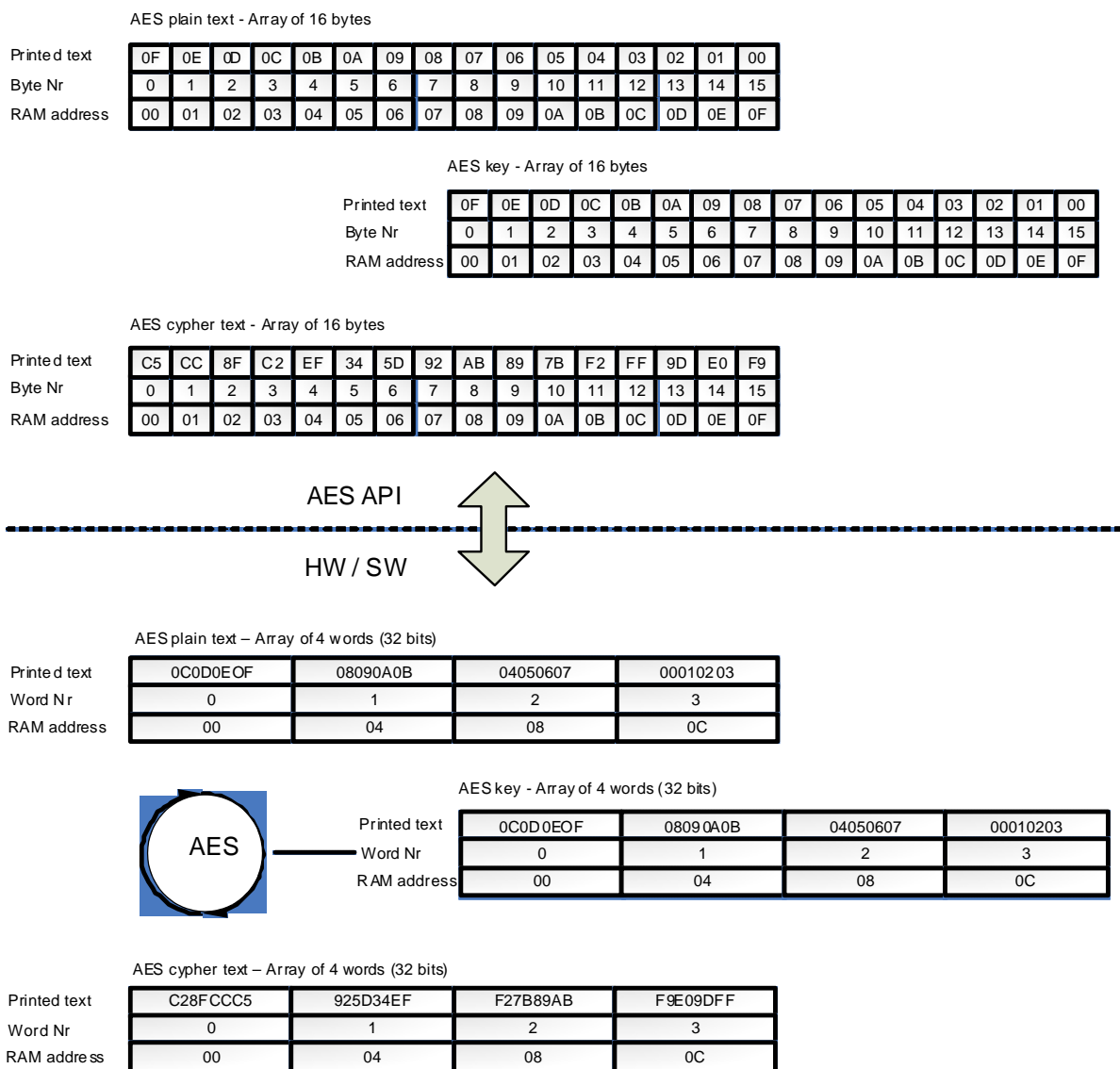
Fig 24. AES endianness
