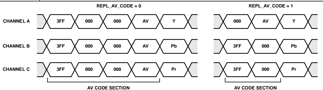
Figure 43. AV Code Output Options (CP)
