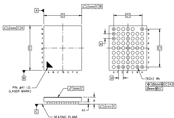
Si4682-A10-GD (WLCSP)
