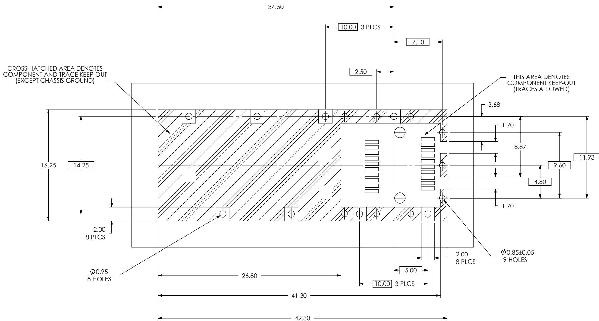
D FIG. 3 (SFPC-SL SHOWN)
