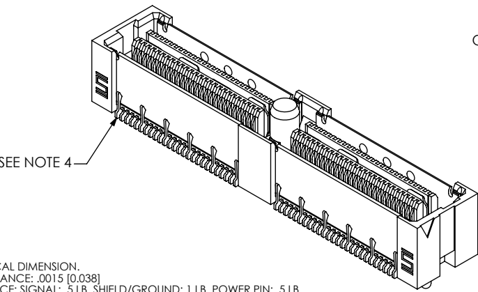
FIG 1 QFSS-052-04.25-X-D-A SHOWN
