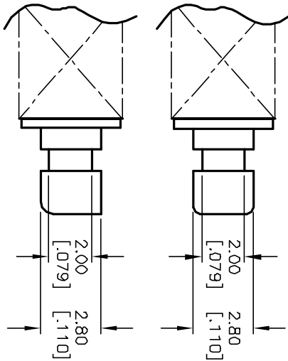
ACTUATOR DETAIL
