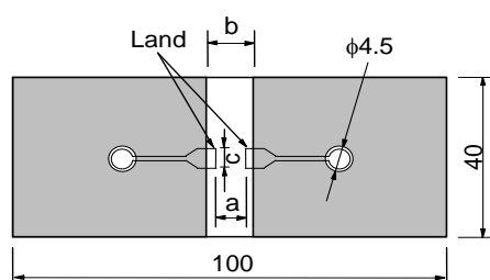
Fig.1 (in:mm)
