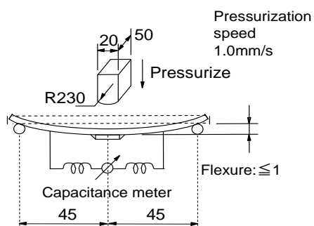
Fig.2 (in:mm)
