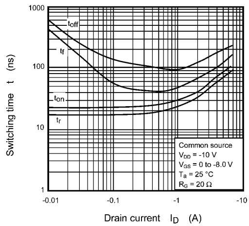
Fig. 7.10 t - I_D
