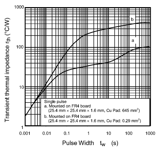
Fig. 7.12 r_{th} - t_w
