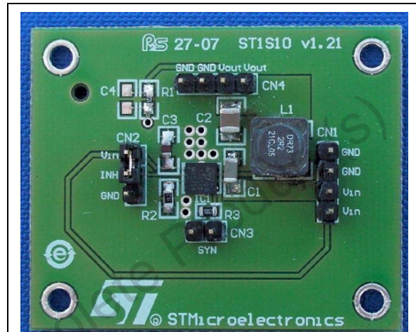
STEVAL-ISA044V2
