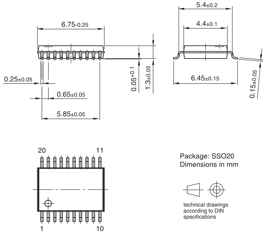
Drawing-No.: 6.543-5056.01-4 Issue: 1; 10.03.04
