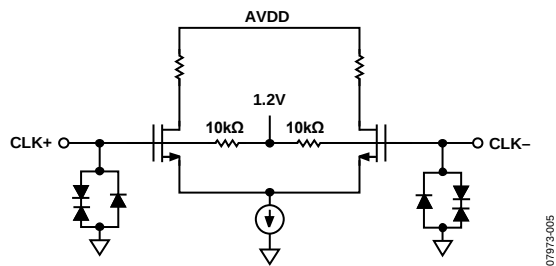
Figure 26. CLK± Inputs
