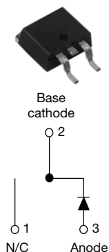
D²PAK
