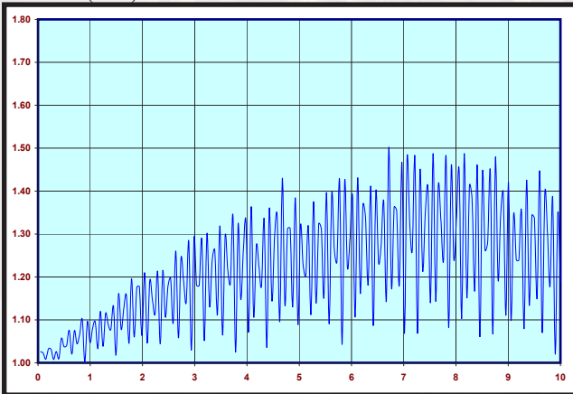
PN: CCSMA-MM-SS402-60 VSWR (S11)
