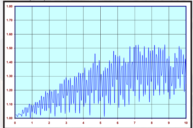
PN: CCSMA-MM-SS402-60 VSWR (S22)
